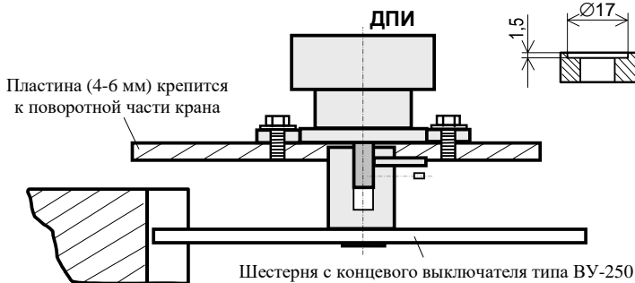
Рисунок 12 – Установка ДПИ
