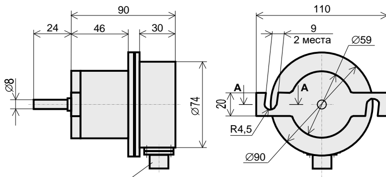
Рисунок 11 – Установка "ДПИ-Ось 360"
