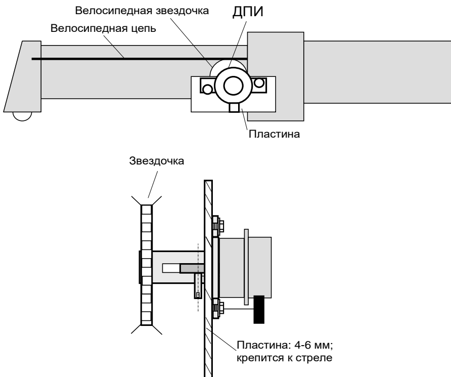
Рисунок 8 – Установка ДПИ (ОНК-160С-32)
