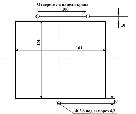
Рисунок 3 – Габаритные и присоединительные размеры БОИ
