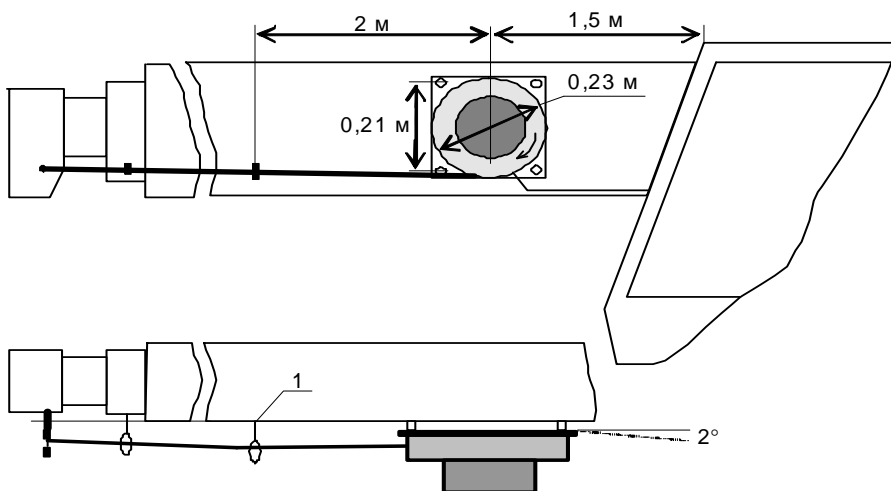
Рисунок 7 – Установка датчиков вылета (ОНК-160С-74)
