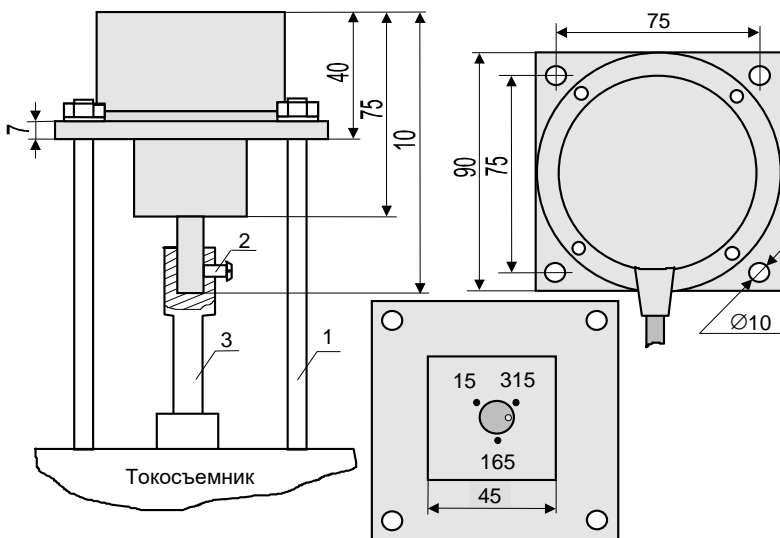
Рисунок 11 – Установка "ДПИ-Ось 360"
