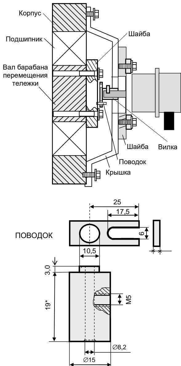
Рисунок 9 – Установка ДПИ (ОНК-160С-31)
